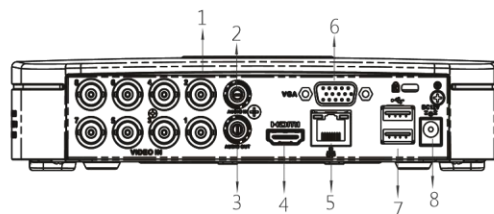
DHI-XVR5108C-S2
