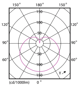
CorePro LEDlustre 40W E14 865 FR P45
