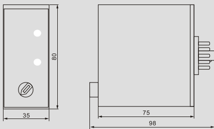
AS-TE101 Outline dimension
