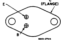
JEDEC TO-3
