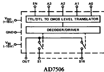
AD7506
