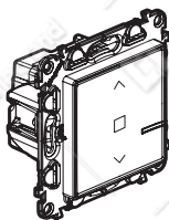
Свързан ключ за щори
