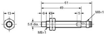
E2A-S08LN04-M5-□□
