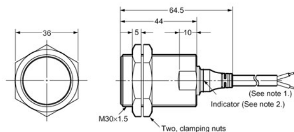
E2A-M30KS15-WP-□□
