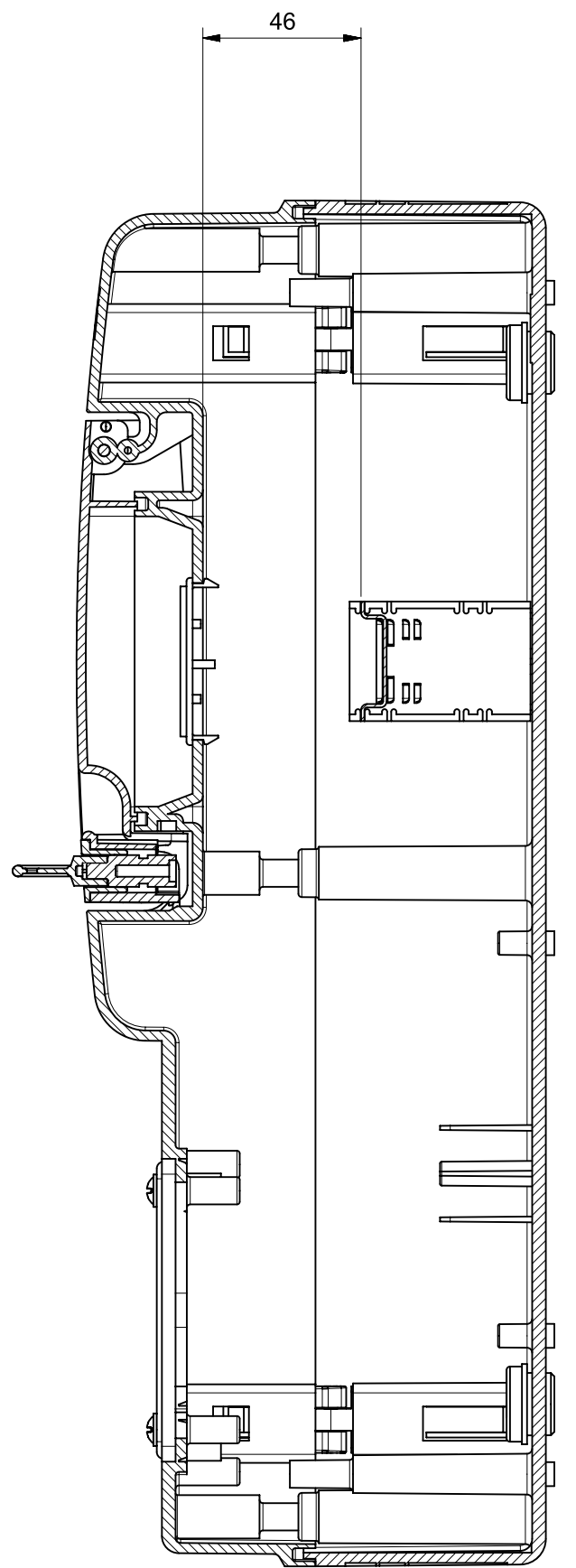
Sezione A-A
