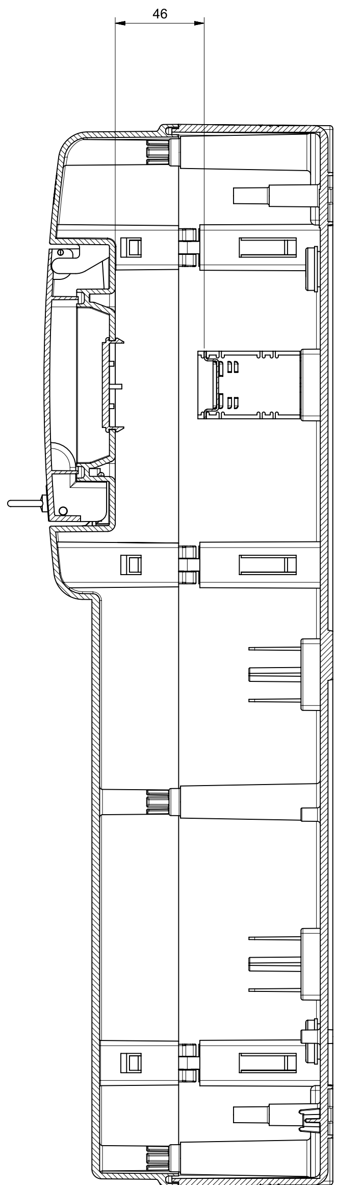
Sezione A-A
