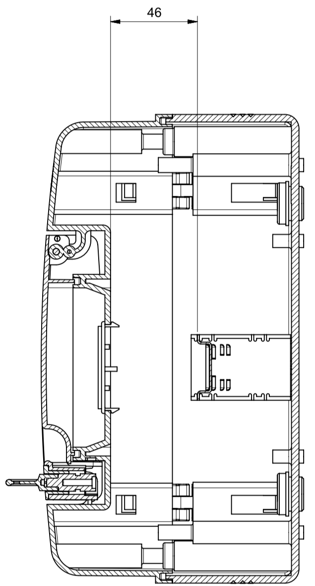
Sezione A-A
