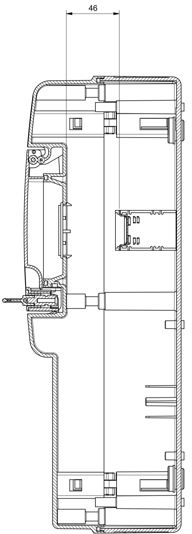
Sezione A-A
