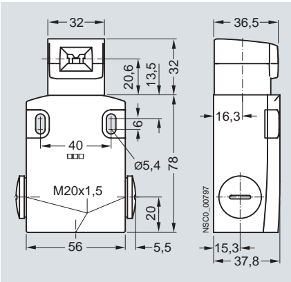
Enclosure width 56 mm 3SE5 12.-.QV10, 3SE5 12.-.RV10
