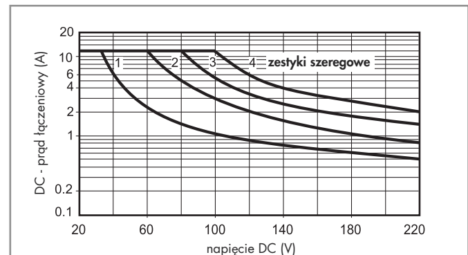
H 56 - Obciążenie graniczne dla prądu stałego (dla DC1) przy obciążeniu rezystancyjnym dla zestyków zwiernych, przerwa estykowa ≥ 1,5 mm
