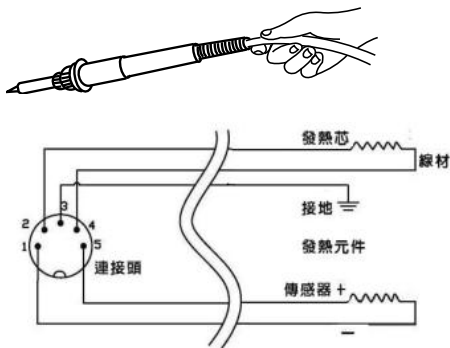
引線示意圖
