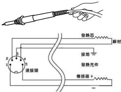
引线示意图
