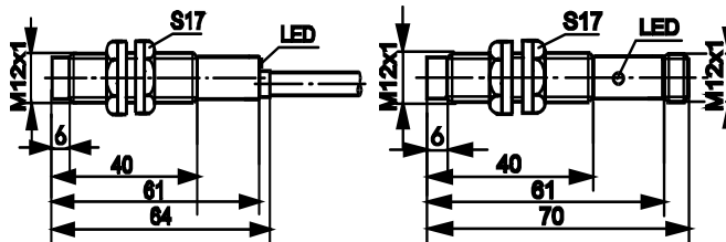
wyjscie kablowe
