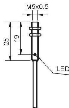
wyjście kablowe / cable output
