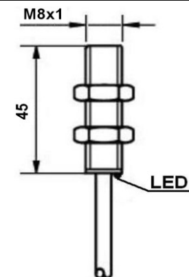
wyjście kablowe / cable output
