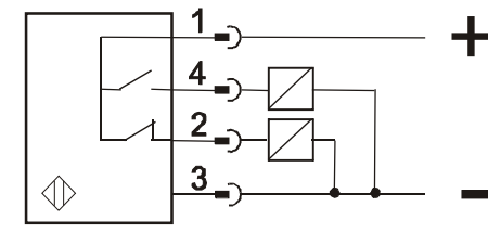
8 PNP/NO+NC
