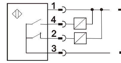
7 NPN/NO+NC
