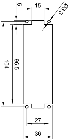
Panel cut out for inserts for use without hood/housing Foratura di alloggiamento inserti per uso senza custodia
