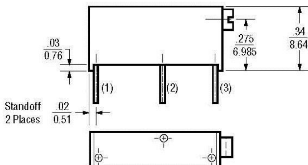
РАЗПОЛОЖЕНИЕ НА ПИНОВЕТЕ 89X
