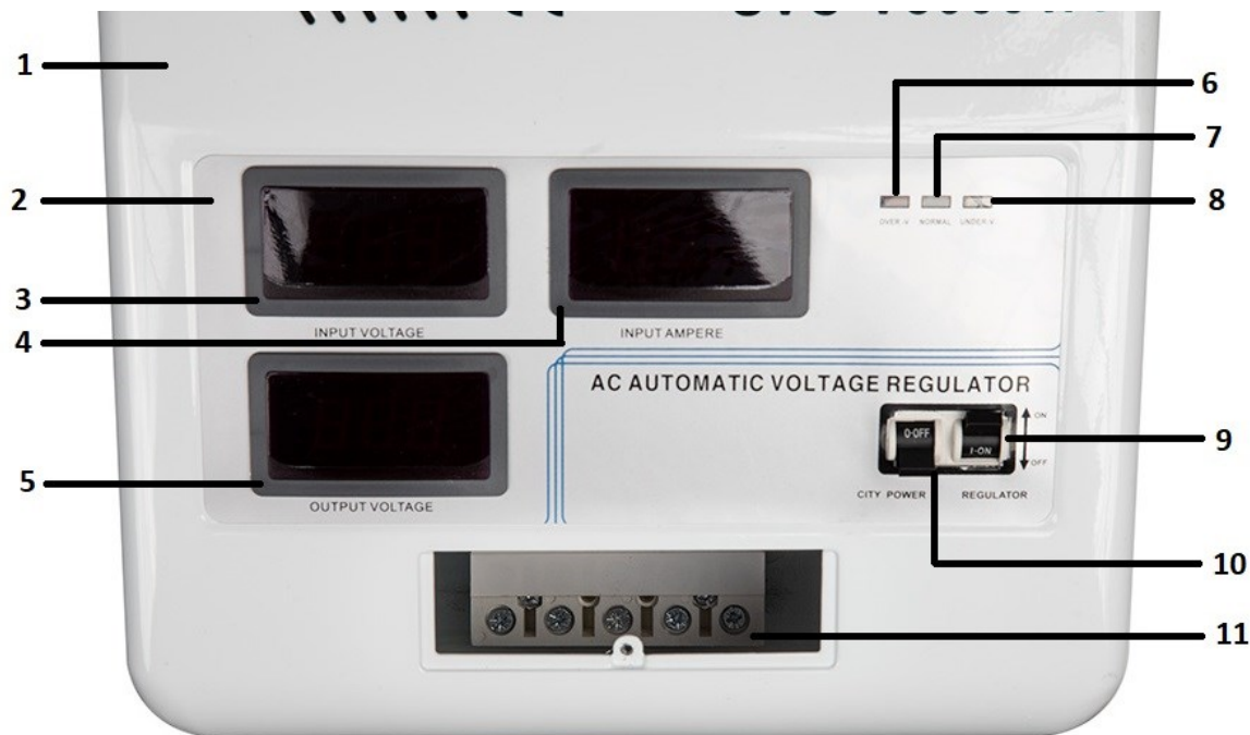
Фигура 3 – Общ изглед на серията SVC-V
