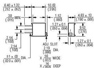
Общи размери
