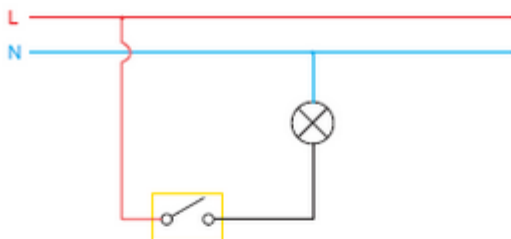
Схема на обикновен ключ
