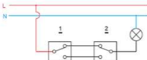
Схема 6 – принципна електрическа схема на свързване на девиаторни електрически ключове, с помощта на която може да се включва и изключва независимо 1 консуматор от 2 точки
