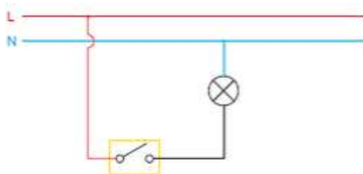
Схема 1 – принципна електрическа схема на свързване на единичен електрически ключ
