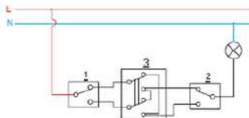
Принципна електрическа схема на свързване на кръстат електрически ключ, с помощта на която може да се включва и изключва независимо 1 консуматор от 3 точки
