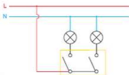
Схема 5 – принципна електрическа схема на свързване на двоен сериен електрически ключ за включване и изключване на 2 вериги
