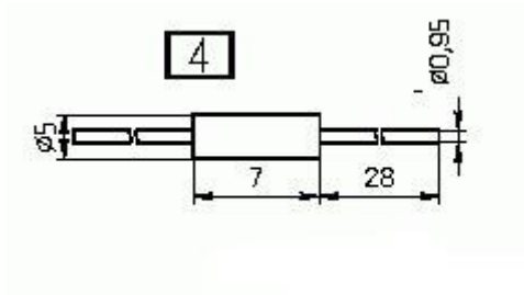
Рисунок 1 - Выпрямительный диод малой мощности КД106А
