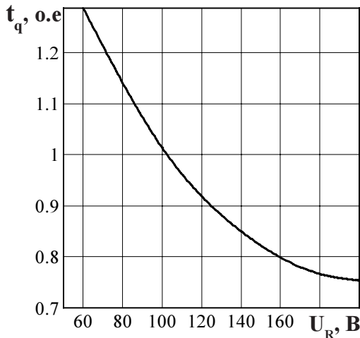
Рисунок 13 - Зависимость времени выключения t_q (о.е.) от обратного напряжения U_R при максимальной температуре перехода T_{jm} = 125^\circ \text{C} ; I_T = I_{T(AV)} ; (di/dt)_f = 5 \text{ А/мкс} ; dU_D/dt = 50 \text{ В/мкс} ; U_D = 0,67 U_{DRM}
