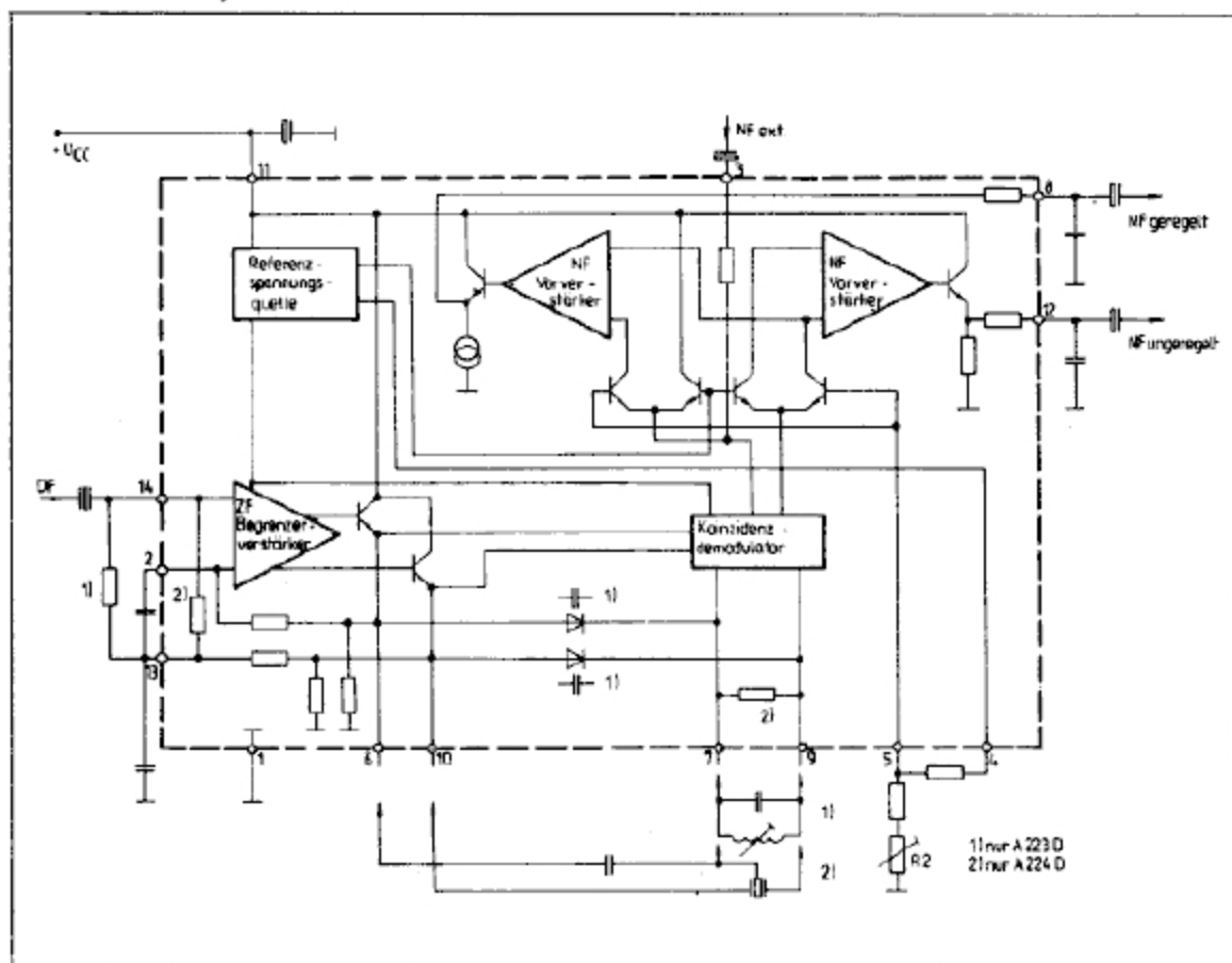
Übersichtsschaltplan
