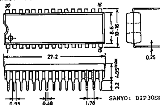
外形図 3061-D30SNIC (unit: mm)
