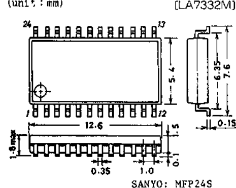
外形図 3112-IC (unit: mm)
